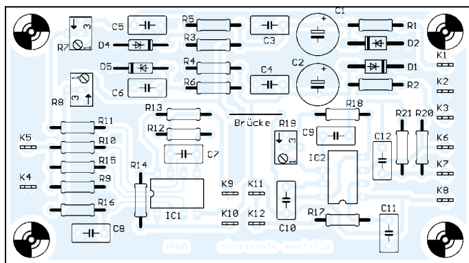
Bild 23: Bestückung der Platine AWP1
