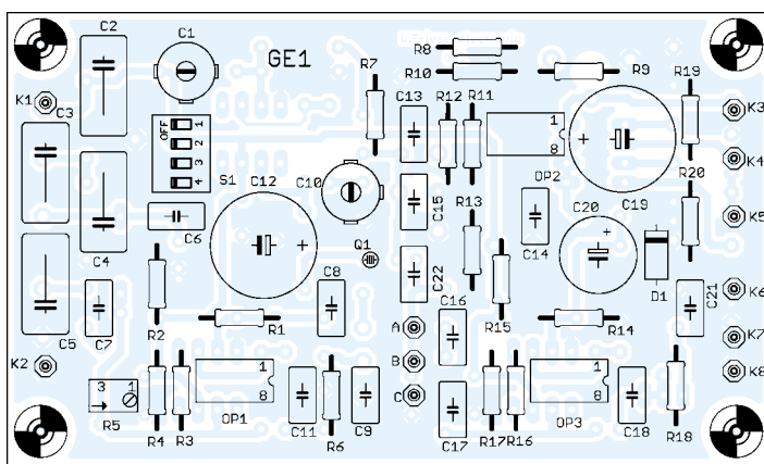
Bild 24: Bestückung der Platine GE1 (oben)
